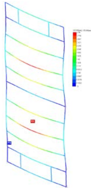
Диаграмма прогибов
